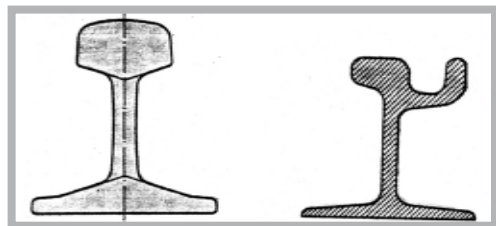
2. ÁBRA A VIGNOL ÉS A VÁLYÚS (PHÖNIX)-SÍN KERESZTMETSZETE
