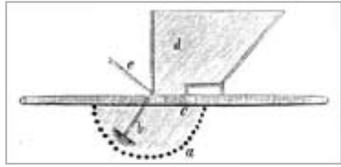
1. ÁBRA EGYSZERŰ SZŐLŐZÚZÓ (BABO-MACH 1893. I. 888.)
