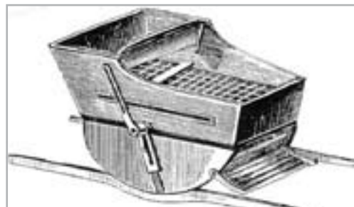
2. ÁBRA ZÚZÓMALOM BOGYÓZÓROSTÁVAL (BABO-MACH 1893. I. 889.)
