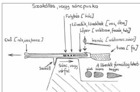
3. MELLÉKLET SZAKÁLLAS VAGY SÁNCPUSKA VÁZLATRAJZA (KÉSZÍTETTE: DANI D. PÁL)
